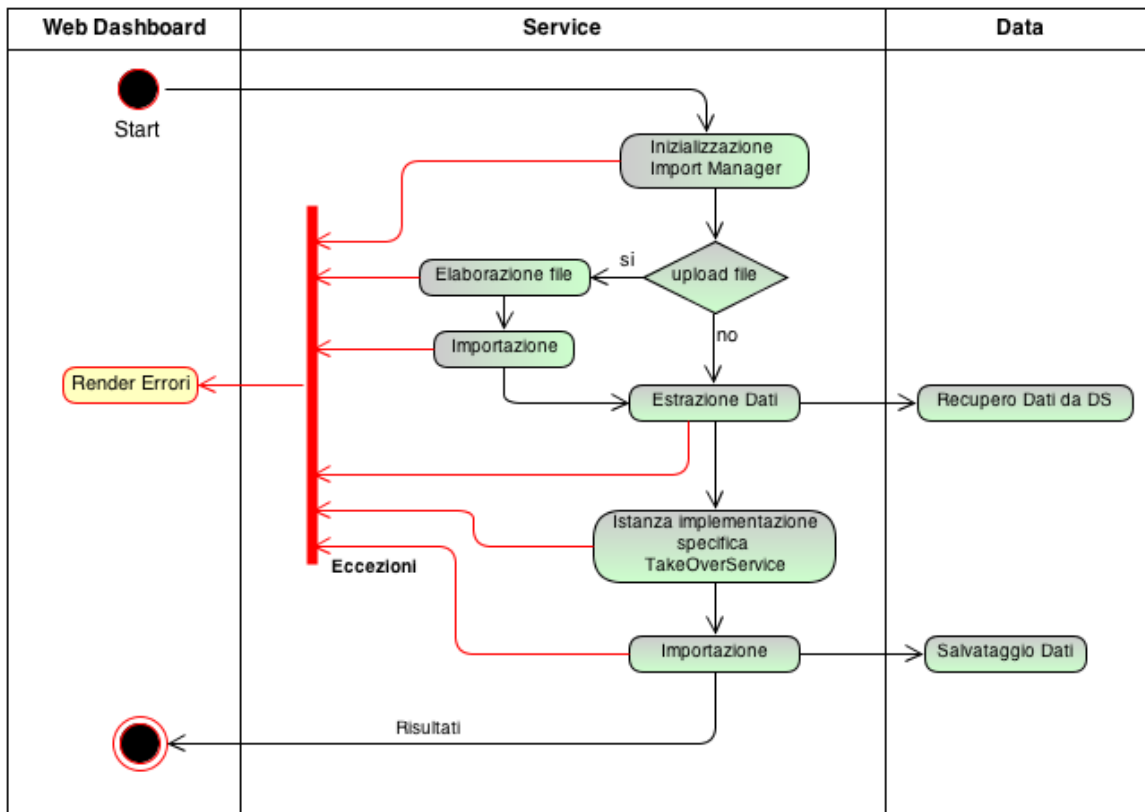
Figura 15 - Activity Diagram del servizio di Interfacciamento Standard
