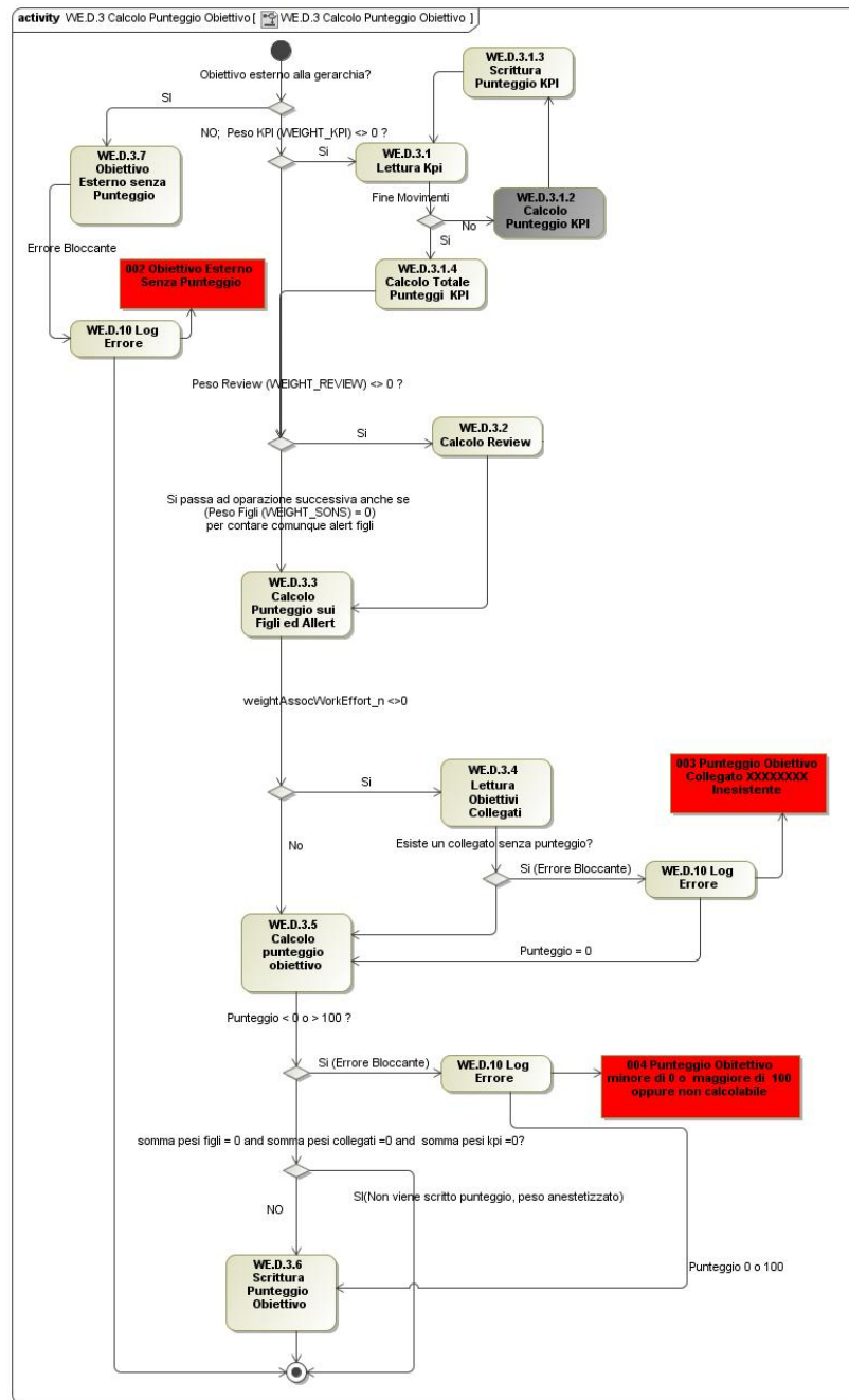
Figura 19 - Algoritmo calcolo punteggio singolo obiettivo
