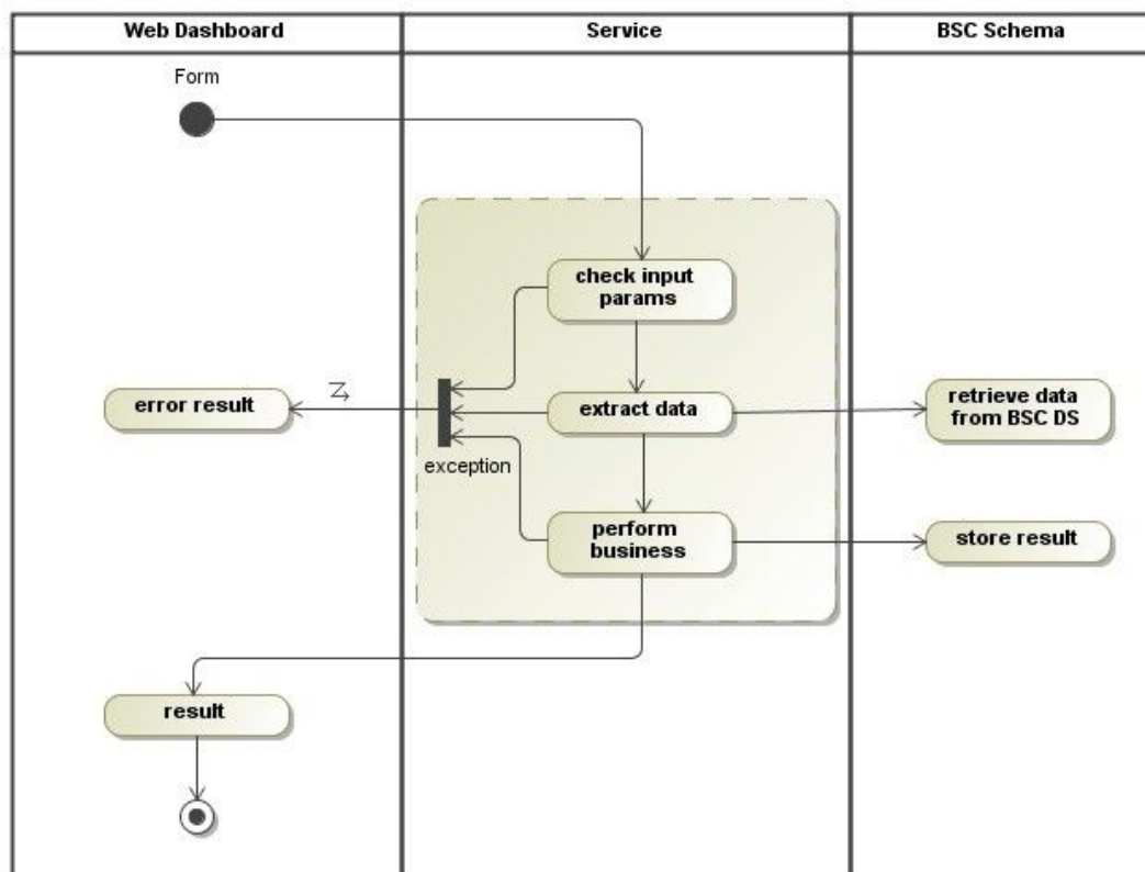
Figura 13 - Richiesta Web Dashboard
