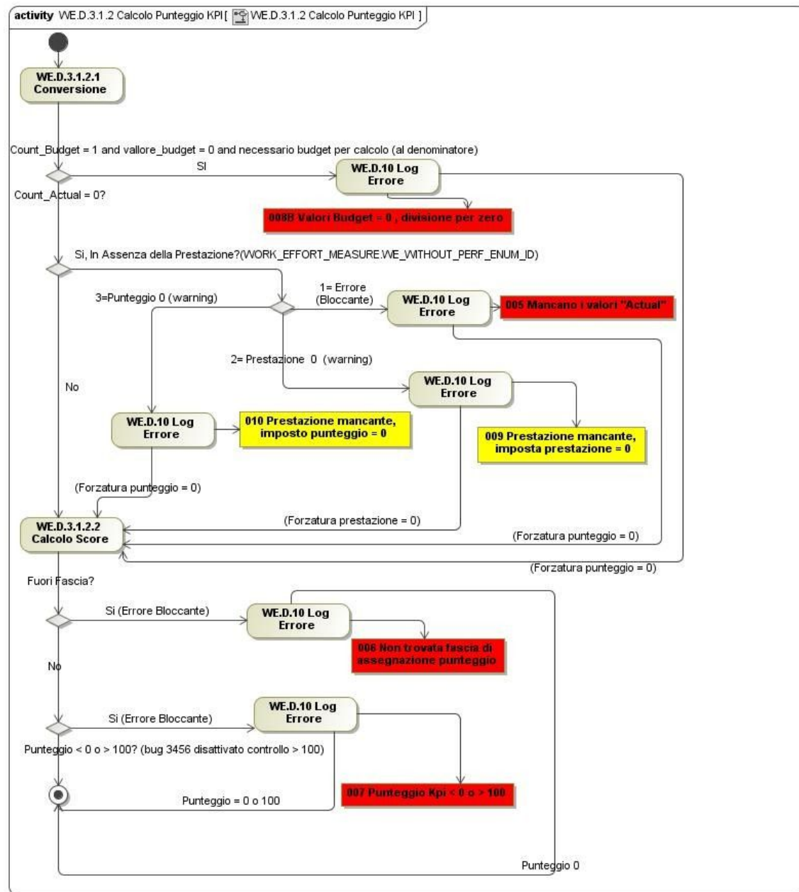
Figura 20 - Algoritmo punteggio KPI
