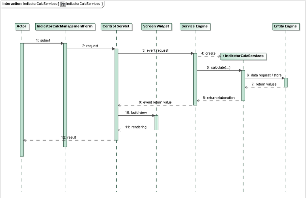
Figura 21 - Sequence Diagram del Calcolo degli Indicatori
