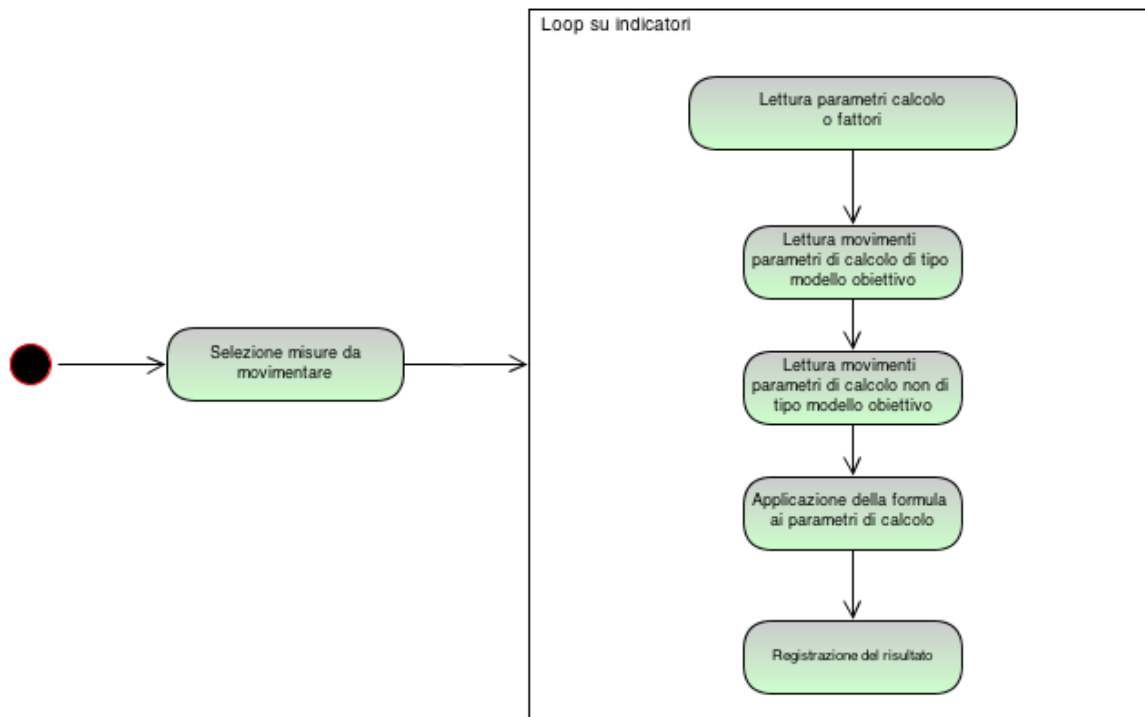
Figura 22 - Activity Diagram per Indicatore modello su obiettivo
