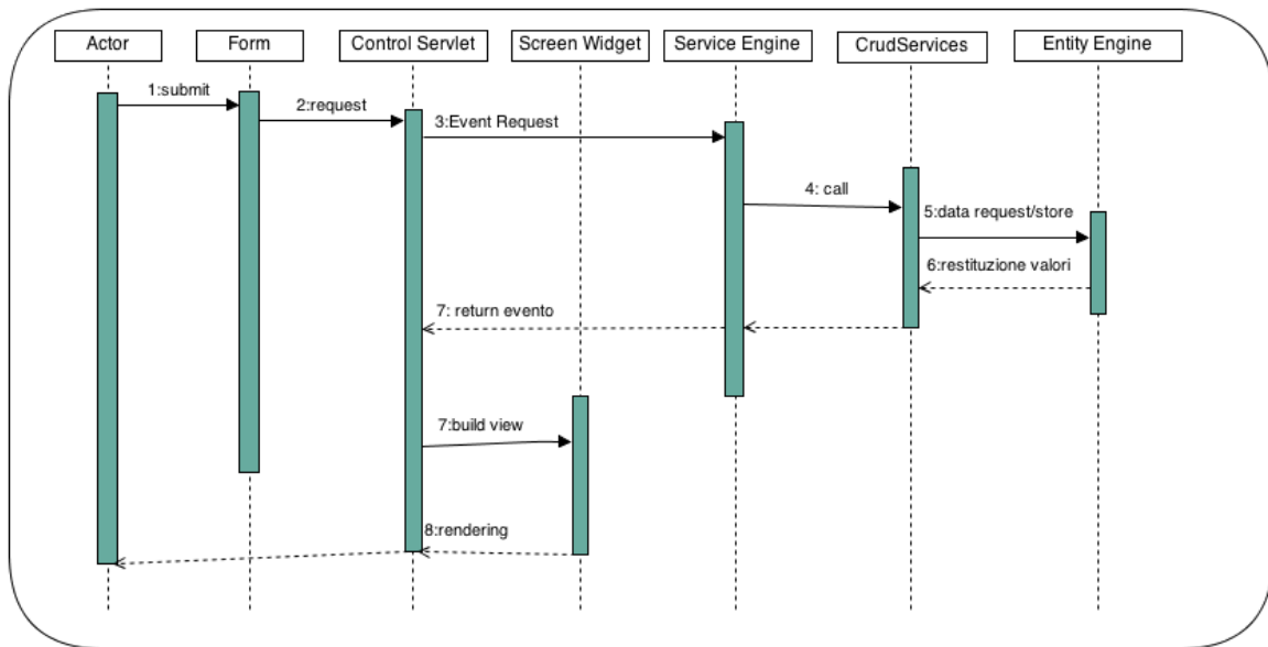
Figura 14 - Sequence diagram Transazioni tra gli stati di un processo
