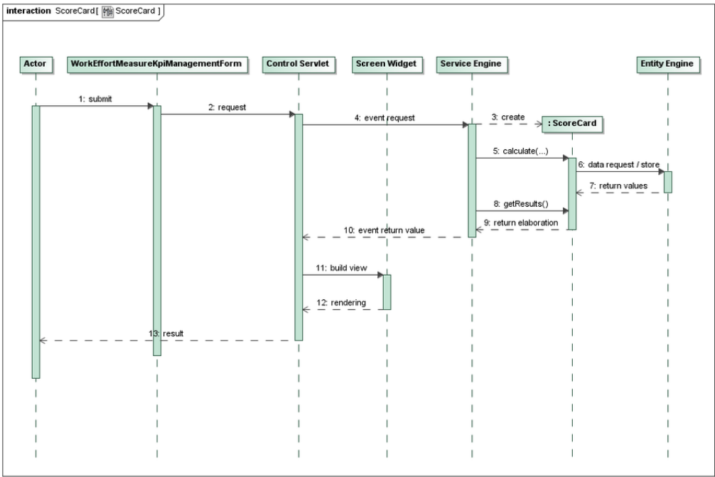
Figura 17 - Sequence Diagram del Calcolo Punteggio
