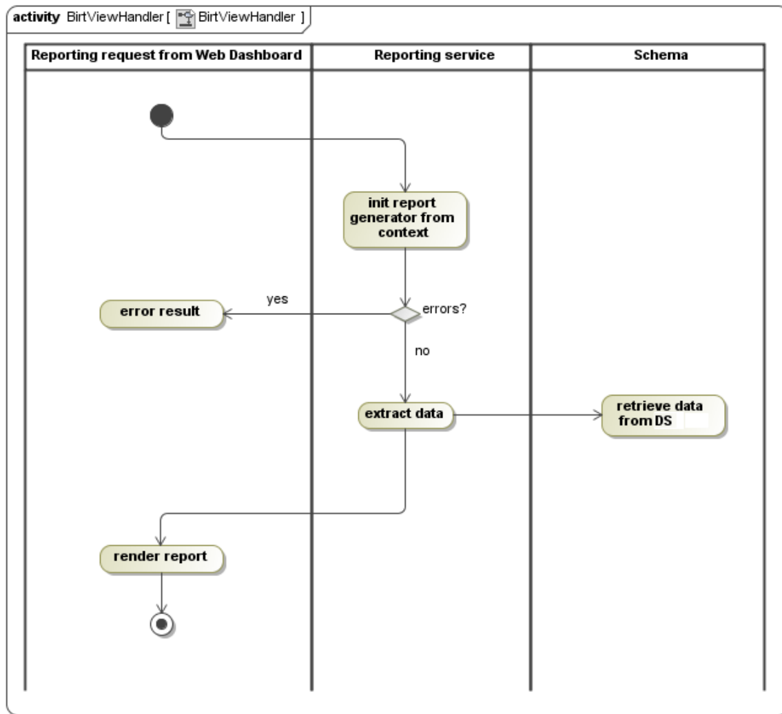
Figura 23 - Activity Diagram del servizio di Reporting
