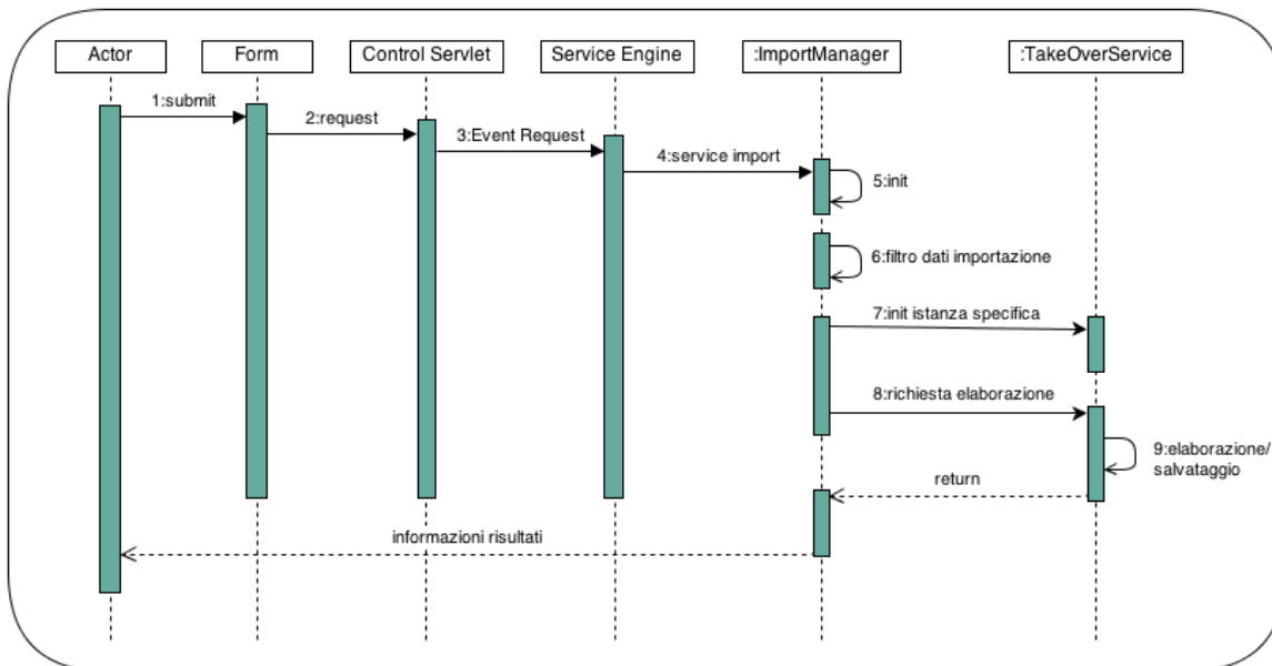
Figura 16 - Sequence Diagram del servizio di Interfacciamento Standard
