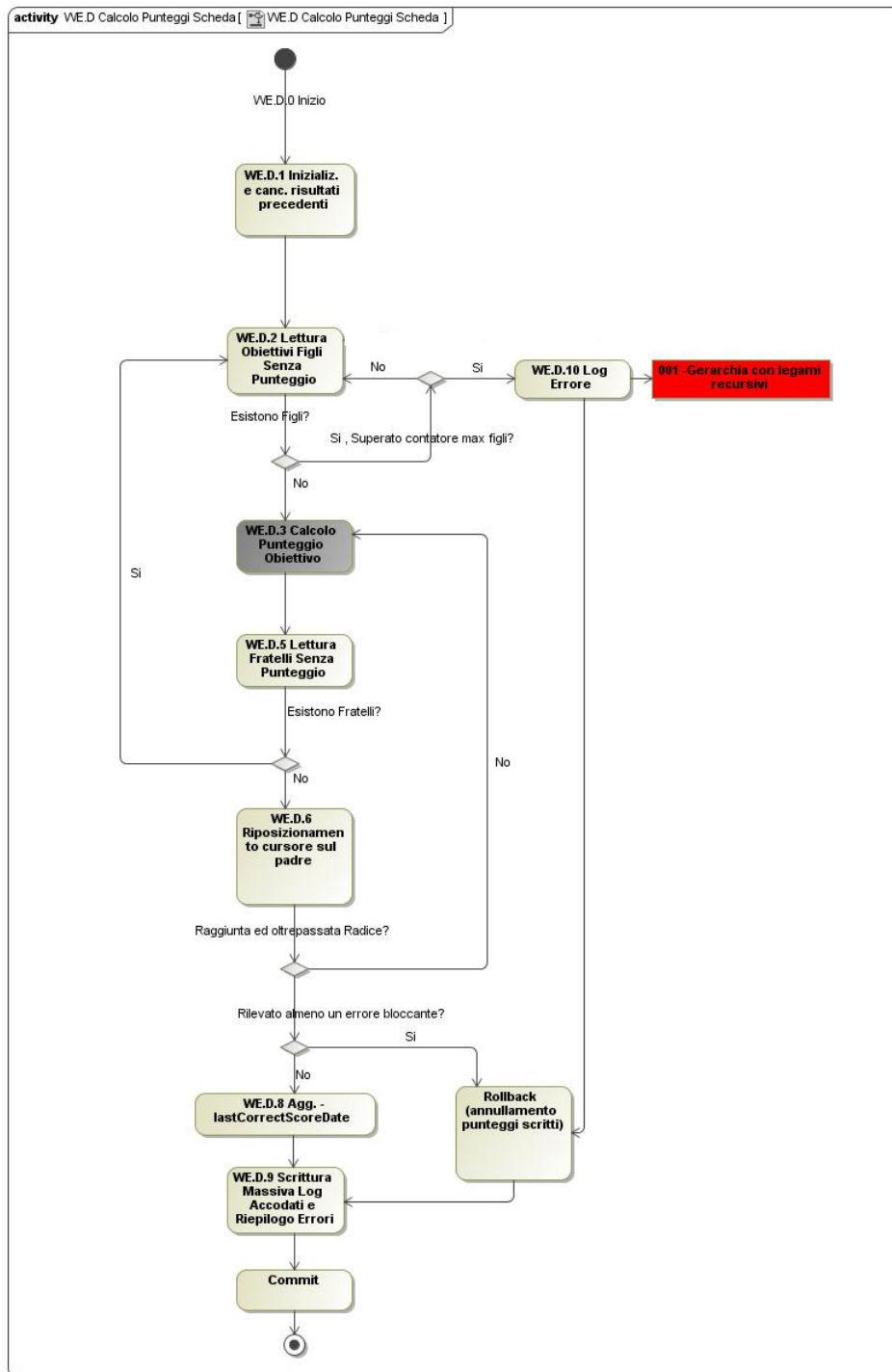
Figura 18 - Algoritmo del calcolo punteggio
